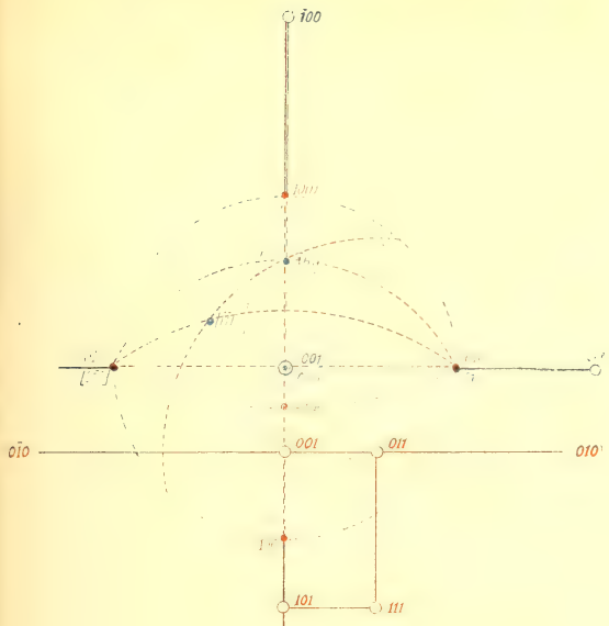
9. Ортопироксенъ.
